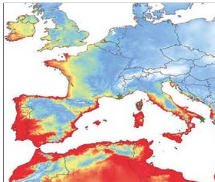
Riesgo de desarrollo de la bacteria en función de las temperaturas mínimas invernales
